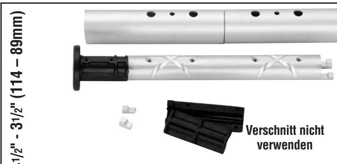
41/2" - 31/2" (114 - 89mm) Oberhalb des obersten Verbinders keine Kunststoff Buchse einsetzen. Verbinder oben kürzen, und Trimmkappe Kürzen, sofern nötig.
