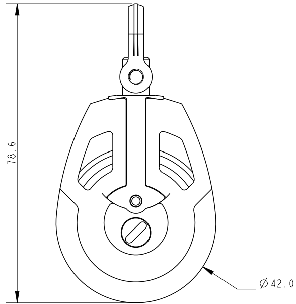
SCALE 1:1
