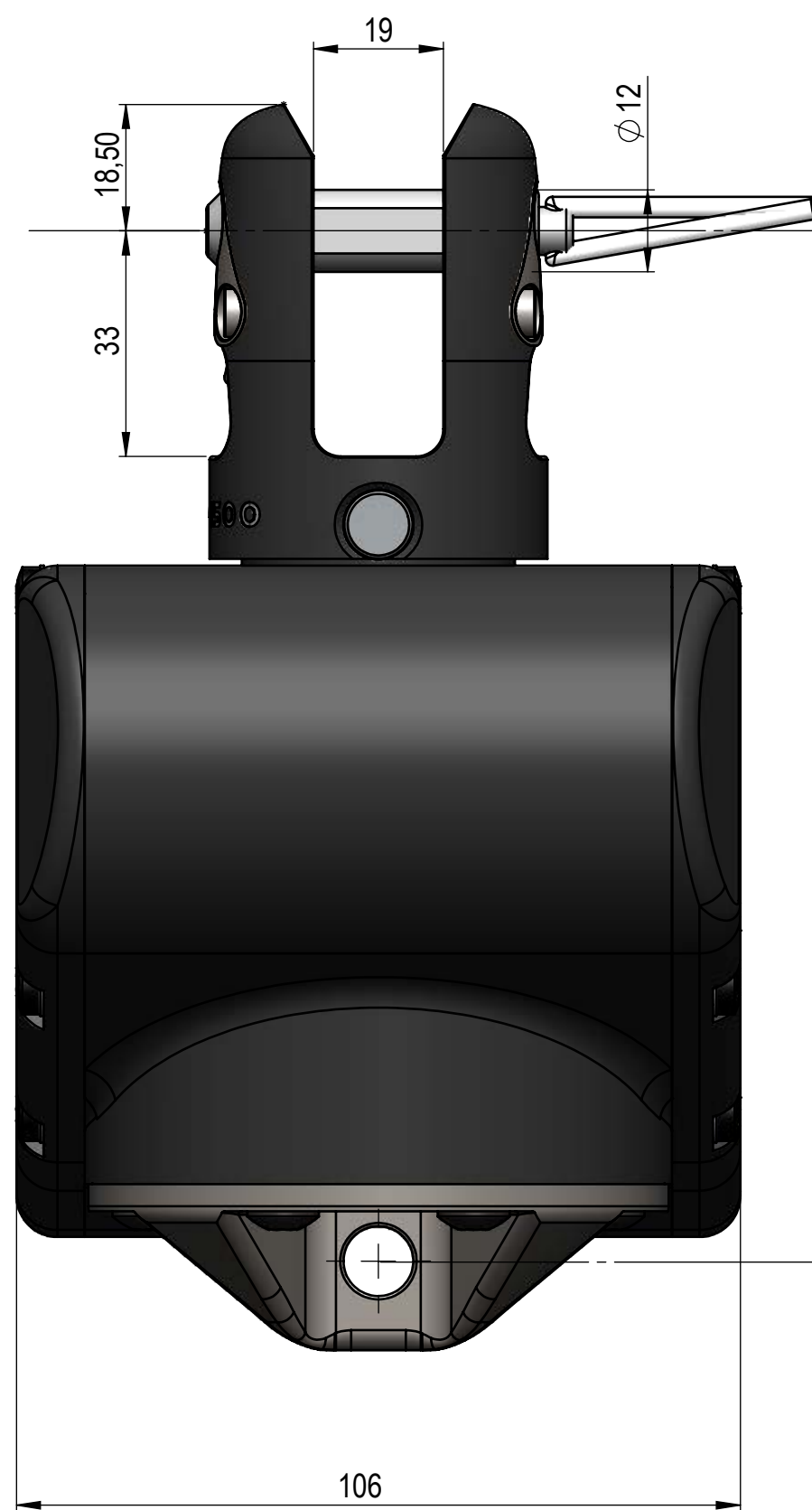
Bloc moteur FXE 4500 électrique / Electric drive unit FXE 4500 43720204530
