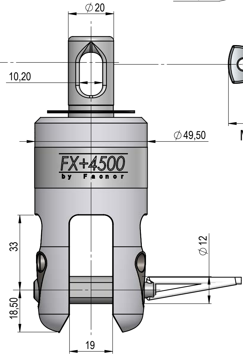
Émerillon FX+ 4500 / FX+ 4500 Swivel 43420104530 Poids / Weight : 493g
