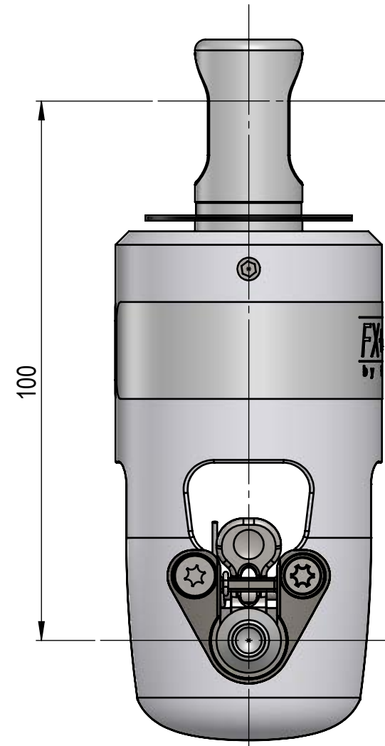
Émerillon FX+ 4500 / FX+ 4500 Swivel 43420104530 Poids / Weight : 493g
