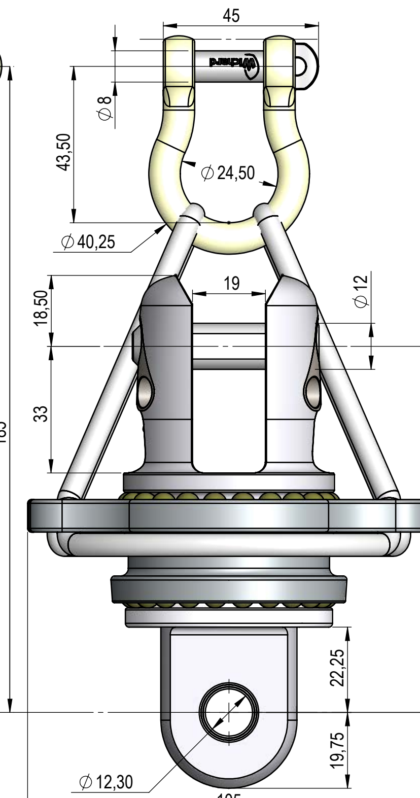
Cosse FAST 4500 / FAST 4500 Thimble 43230004540 (Fournie avec Loop / Supplied with Loop) Poids / Weight : 584g
